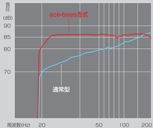
● 通常のアンプ内蔵のサブウーファーと「ace-bass」方式サブウーファーの周波数特性の比較
